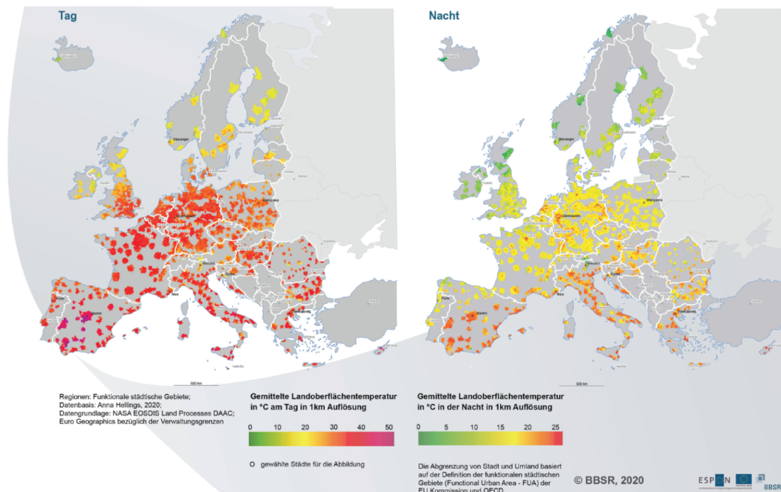
Abb. 5: Durchschnittliche Temperatur in Stadt und Umland 01.-14. August 2020
